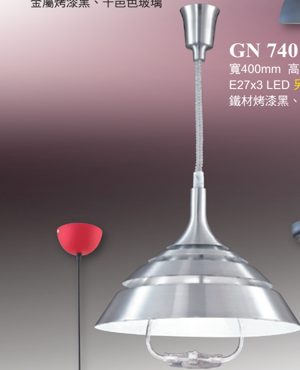
GN 74015 ( 35000 ) 寬450mm 高390mm 線長300~600mm E27x1 LED 另計 鋁製品、附ON/OFF開關
