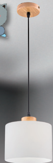
GN 74001 ( 13800 ) 寬180mm 高160mm 線長1000mm E27x1 LED 另計 金屬仿木烤漆、原木、大圓玻璃
